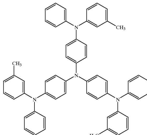
m-MTDATA
